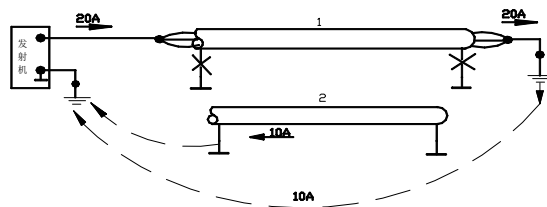
图 7 将电缆屏蔽层与系统地断开
