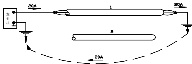
图 8 通过地钉的回电路
