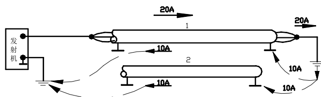
图 6 两根电缆的差值场
