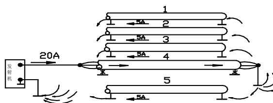
图 5 差值场
