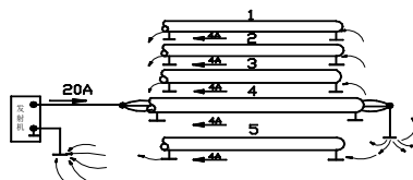
图 4 返回电流的分配
